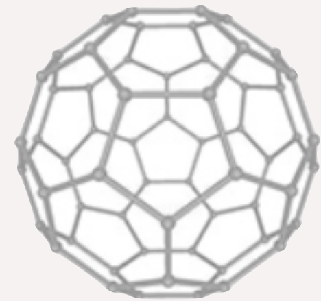
структура углерода
